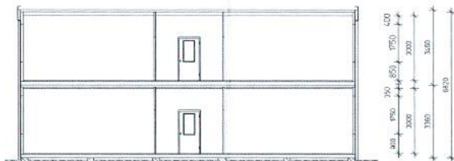
Schnitt E-E
